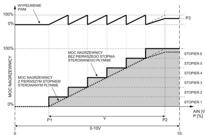
Rys. 5. Schemat pracy CHE2 z nagrzewnicą elektryczną 6-stopniową
