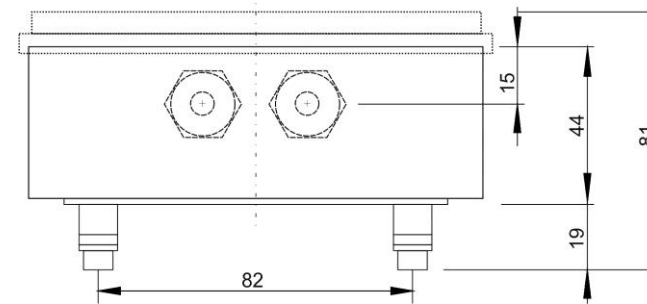
Rys. 8. Wymiary układu CHE2 w obudowie
