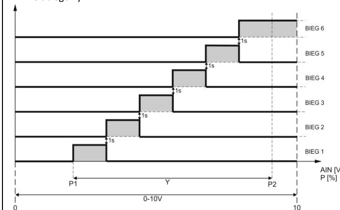
Rys. 6. Schemat pracy CHE2 z silnikiem wielobiegowym
