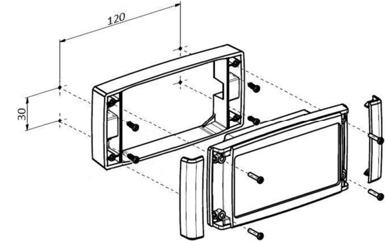
Rys. 3. Montaż natynkowy:
