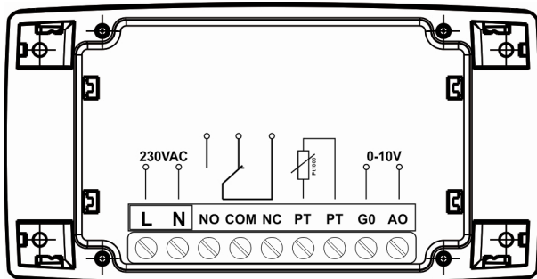
Rys. 5. Listwa opisowa
