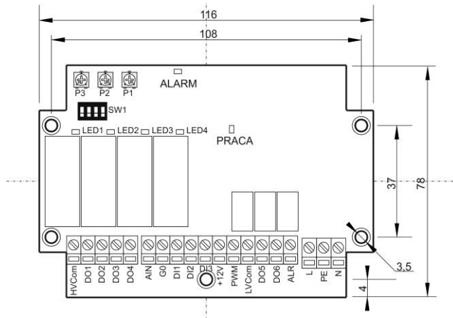
Rys. 7. Płyta elektroniczna CHE2
