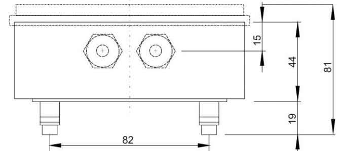
Rys. 8. Wymiary układu CHE2 w obudowie
