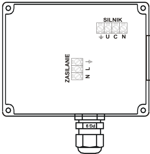
Rys. 2. Zaciski połączeniowe regulatora
