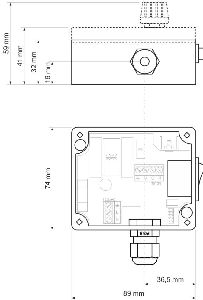
Rys. 4. Wymiary obudowy regulatora DSS2 T-1,5
